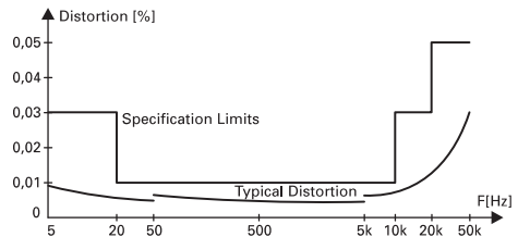
Klirrfaktorverlauf in Abhängigkeit von der Frequenz
